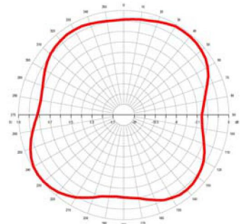
H-Plane
